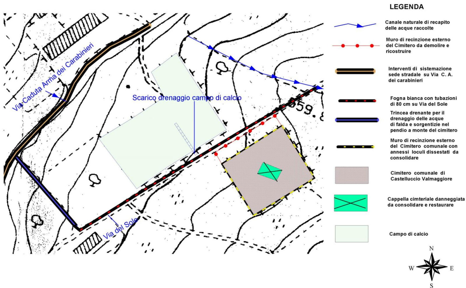
Figura 2. Schizzo planimetrico con indicazione degli interventi in località "Zona Cimitero"
