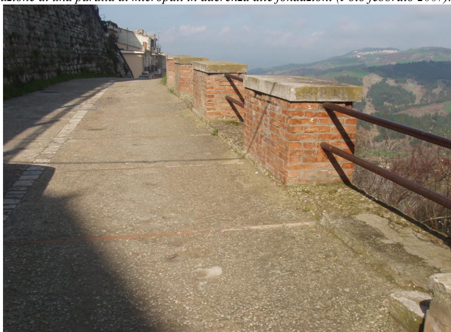
Figura 16. Intervento Zona “F”: Via Fratelli Bandiera – Panoramica della zona interessata dai lavori di consolidamento dei fabbricati e della sede stradale tramite l’esecuzione di paratie di micropali e opere idrauliche per la regimazione e smaltimento delle acque meteoriche (Foto febbraio 2007).
