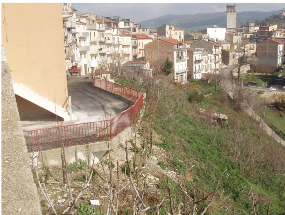
Figura 19. Intervento Zona "H": Consolidamento in Via Carab. Attilio Armando Lombardi: Panoramica della zona a lavori ultimati (Foto febbraio 2007).
