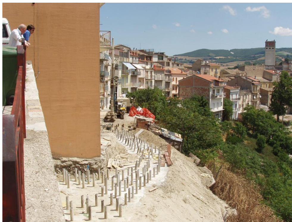
Figura 18. Intervento Zona “H”: Consolidamento in Via Carab. Attilio Armando Lombardi: Paratia di micropali nel pendio sotto i fabbricati in fase d’esecuzione (Foto giugno 2005).
